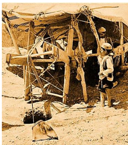
شکل ۴- تصویری از میله چاه قنات و فرآیند لایروبی و خروج گل و لای انباشته شده کوره قنات (ؤلف ۱۹۶۸).
