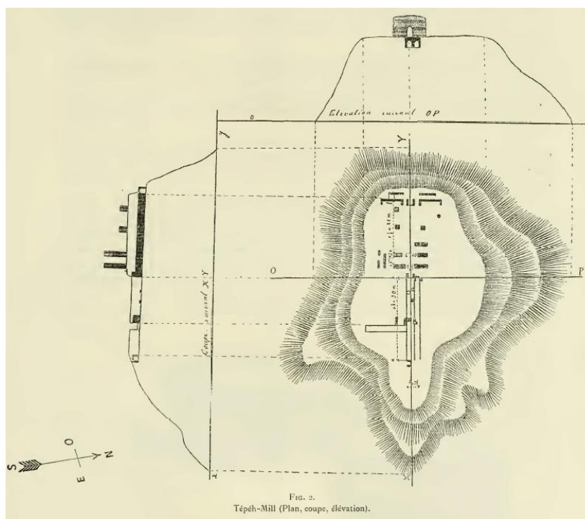
تصویر ۱۲. پلان و مقطع تپه میل (Pézard and Bondoux 1911: 53, Fig. 2).
