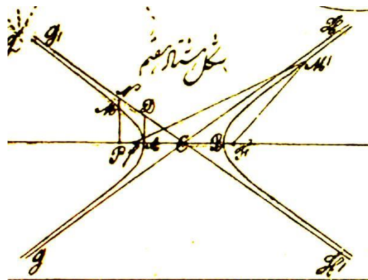
تصویر ۳، هیپربول
